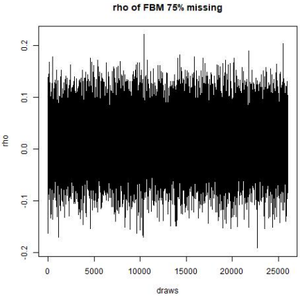
(d) 75% Missingness
